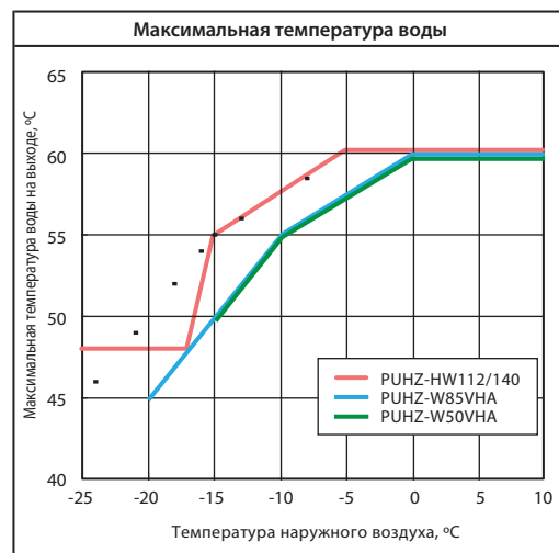
Встроенный теплообменник PUHZ-HW112, 140VNA / YNA2
