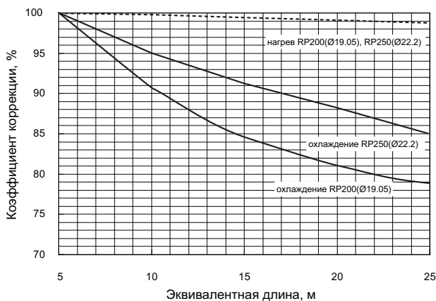
3) График 3. Диаметр газовой трубы на 2 типоразмера меньше стандартного значения.
