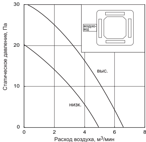
● 4 потока (заслонка - горизонтально). Прямоугольный воздуховод.
