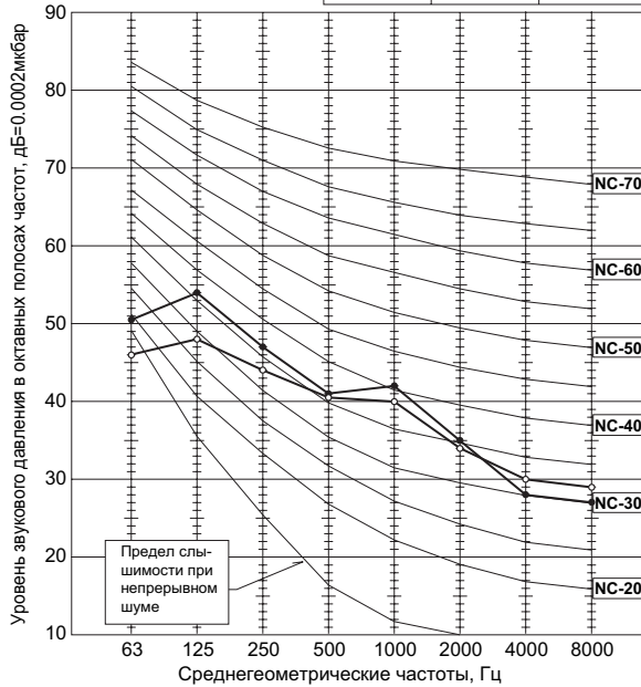
PUHZ-RP35VHA2 PUHZ-RP50VHA2
