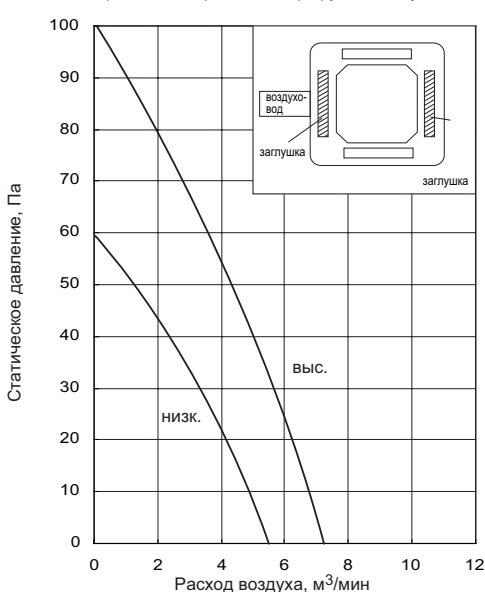
● 2 потока (заслонка - горизонтально). Круглый воздуховод.
