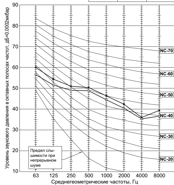
PUHZ-RP125/140VHA2 PUHZ-RP125/140YHA2
