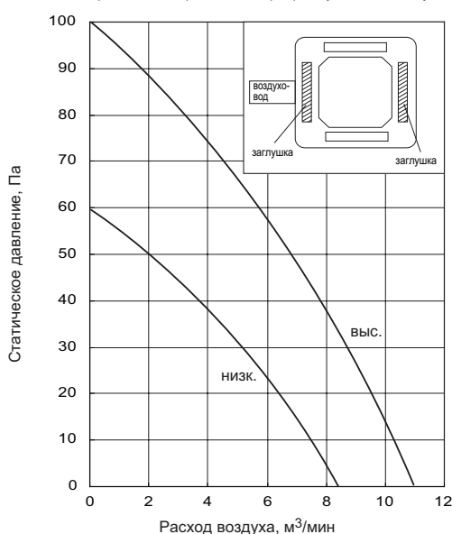
● 2 потока (заслонка - горизонтально). Прямоугольный воздуховод.
