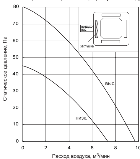
● 3 потока (заслонка - горизонтально). Прямоугольный воздуховод.
