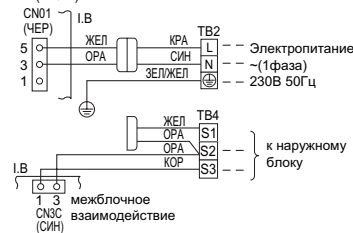
*1 (Рис. 1)
