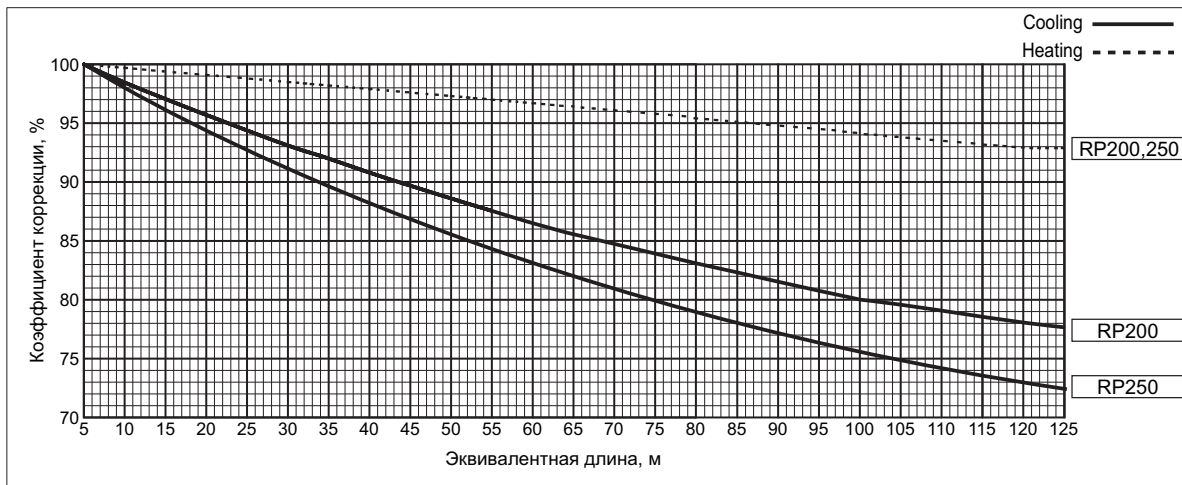
1) График 1. Диаметр газовой трубы имеет стандартный типоразмер.
