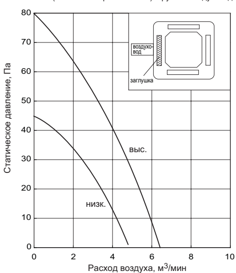
● 3 потока (заслонка - горизонтально). Круглый воздуховод.
